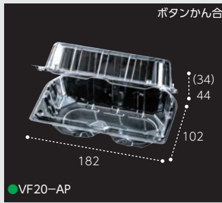
●VF20-AP
