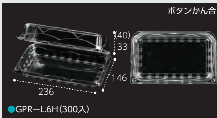
●GPR-L.6H(300入)
