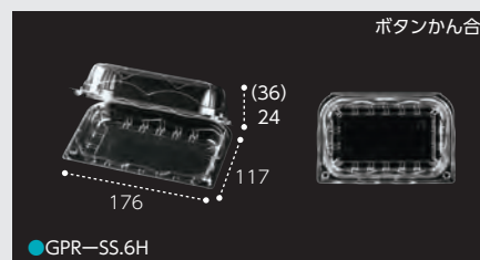
●GPR-SS.6H
