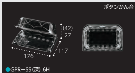
●GPR-SS(深).6H
