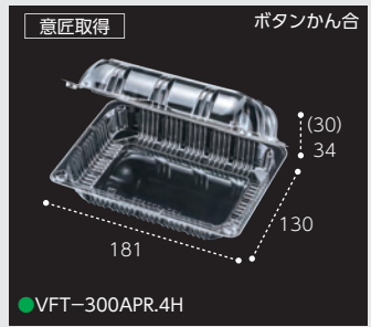
●VFT-300APR.4H
