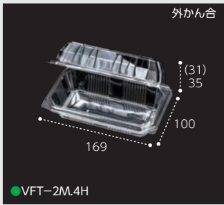
●VFT-2M.4H
