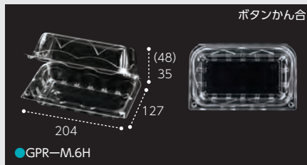
●GPR-M.6H
