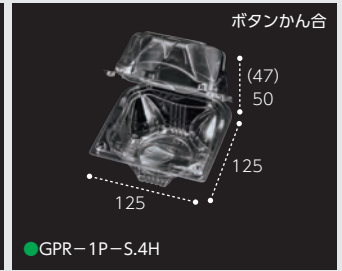
●GPR-1P-S.4H
