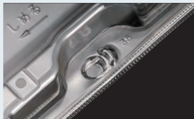
スライドかん合の突起部分 (写真は裏側から撮影)
