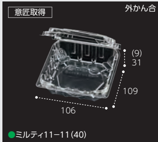
●ミルティ11-11(40)
