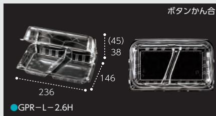
●GPR-L-2.6H
